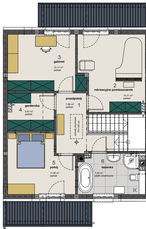
Rzut poddasza
